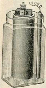
Pile au sel ammoniac, qualité supérieure, vase poreux et verres paraffinés.
